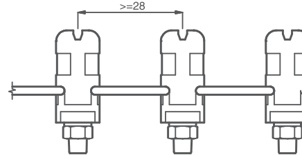
Technische Zeichnung HE
